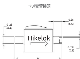
Tube 對焊
