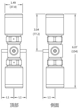
多閥歧管
