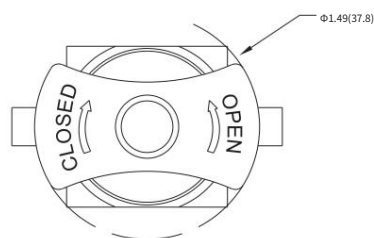
定向手柄
