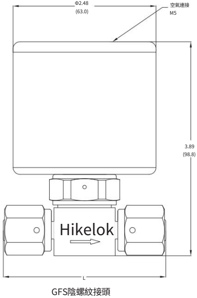
氣動執行器
