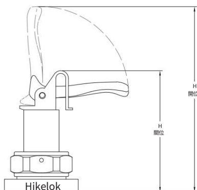
撥動手把
