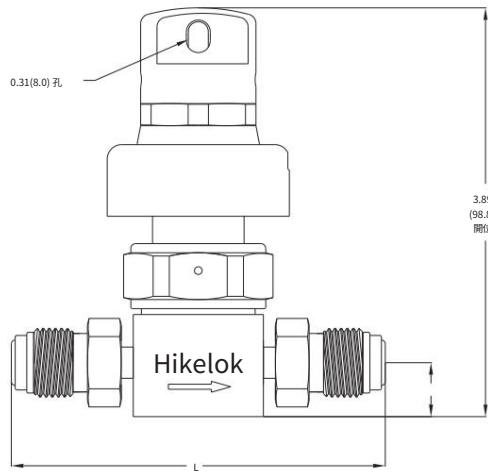
可旋轉GFS陽螺紋接頭
