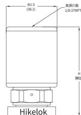
氣動執行器
