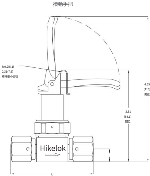
GFS陰螺紋接頭
