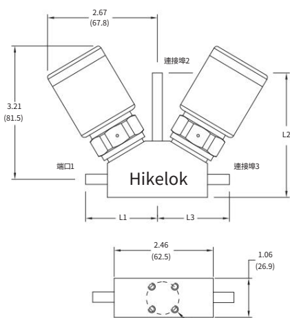
V型和W型多閥閥組
