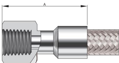
NPT陰螺紋
